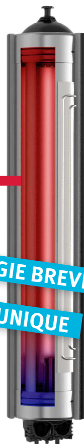
Ballon de 3,2 litres intégré à la chaudière
