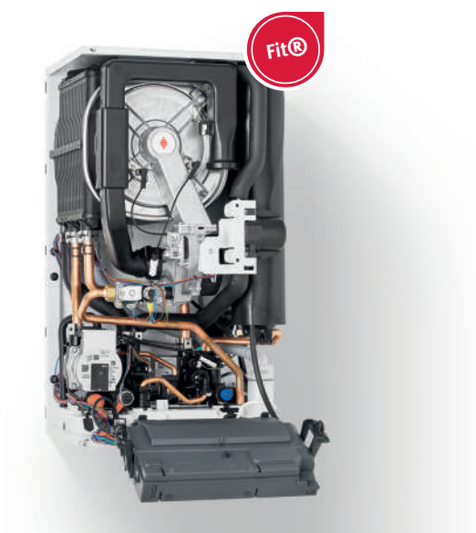
Vue intérieure ThemaPlus H-Condens
